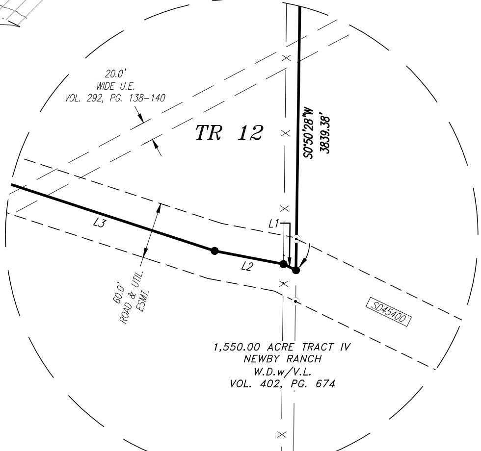
INSET "A" SCALE: 1"=100'
